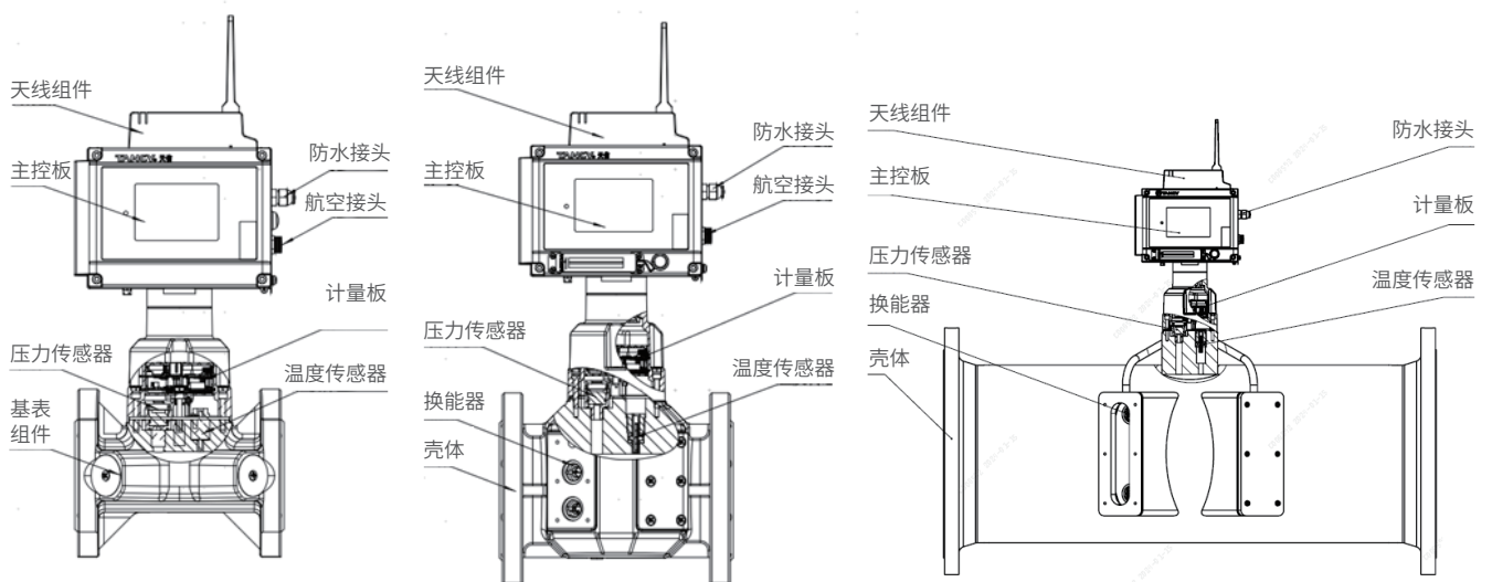
图 3-4 流量计结构图
