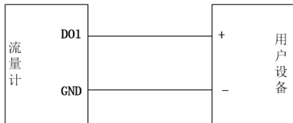
图 6-26 数字量报警信号连接
