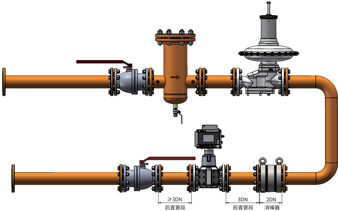
图 5-9 DN150~DN200 安装方式 (调压器后 + 消噪器)
