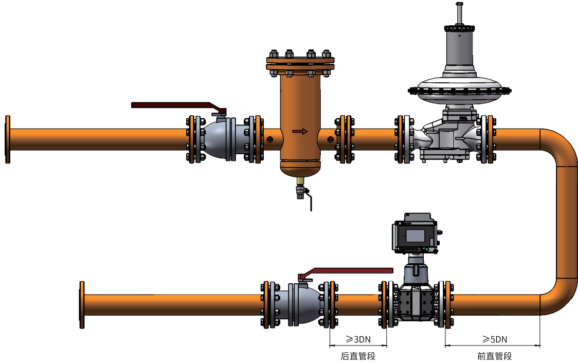
图 5-8 DN25~DN100 安装方式 (调压器后)
