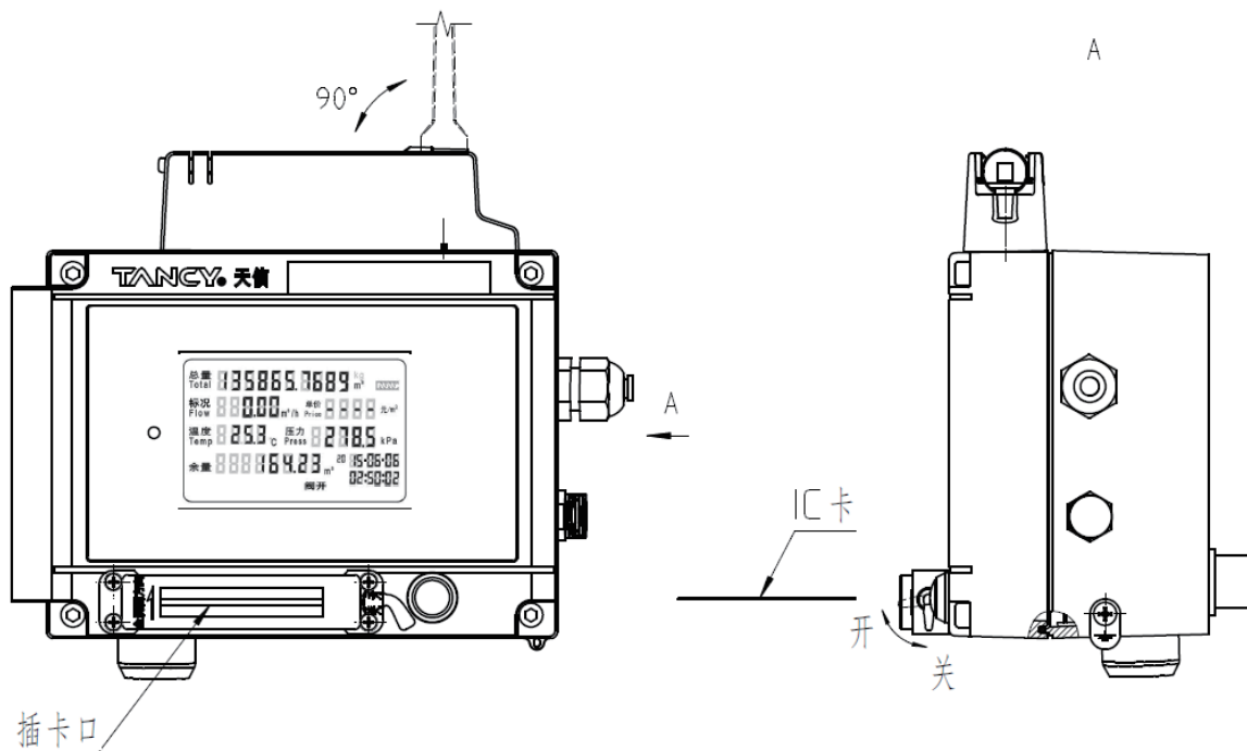
图 6-16 插卡示意图
