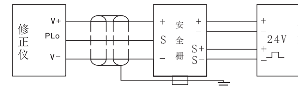
图9 脉冲输出（安全栅可选GS8052）
