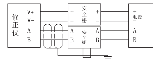
图10 RS485通信（安全栅可选GS8093）
